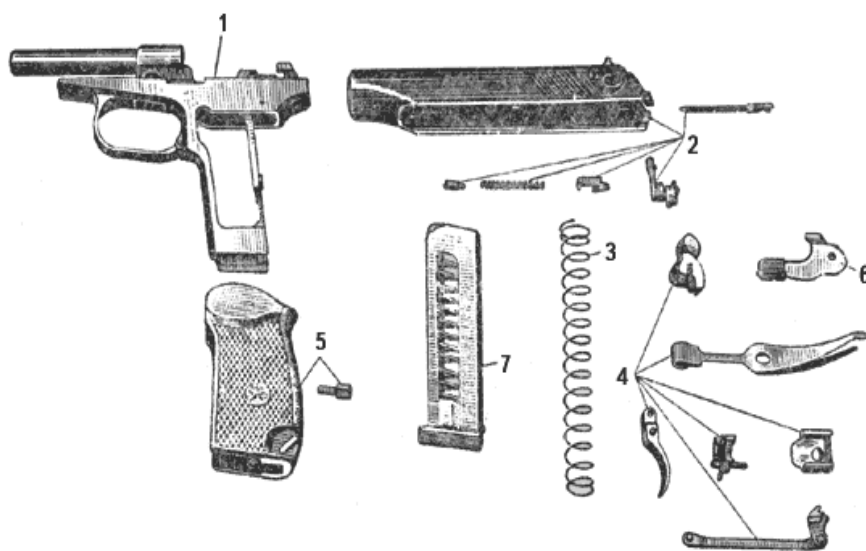
9 мм. тапанша патронының құрылғысы
