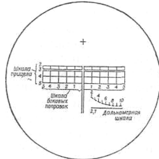
11-сурет. Оптикалық көздеуіш торы
