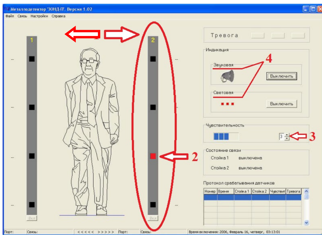
Рис. 4. Изображение экрана металлодетектора «Зонд-П»:
