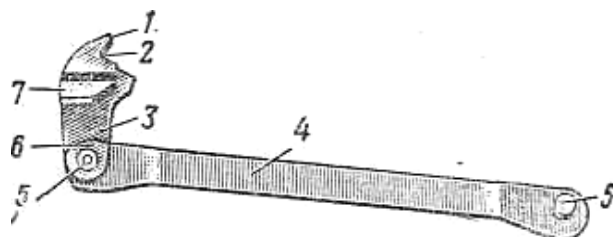
Ағытқышты тартушы иінтірек взводымен
