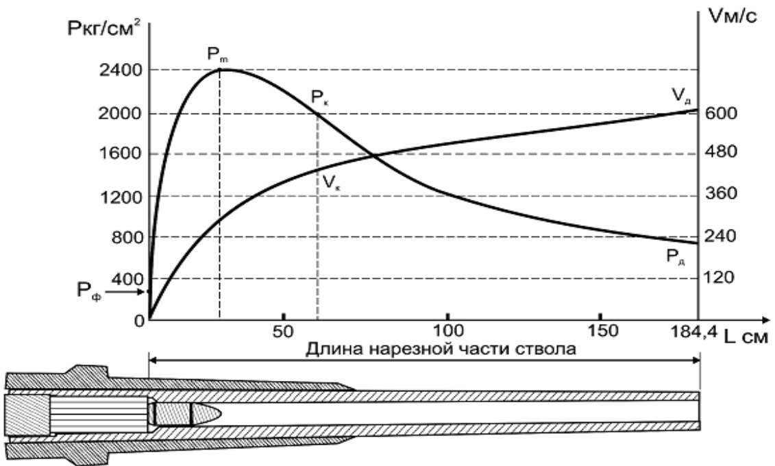
График изменения давления газов и скорости снаряда в стволе в зависимости от пути.
