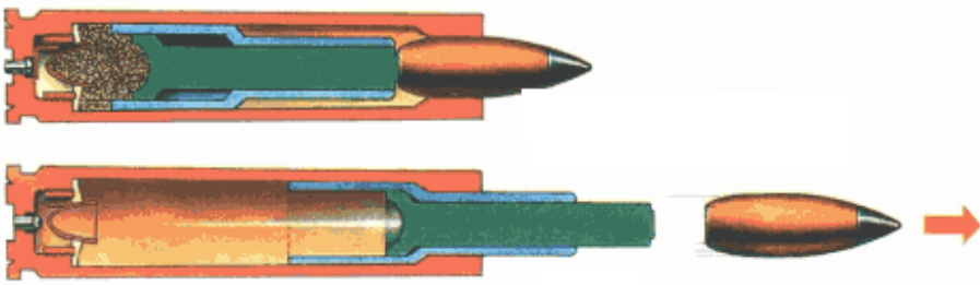
Рис. 4. Патрон СП-3
