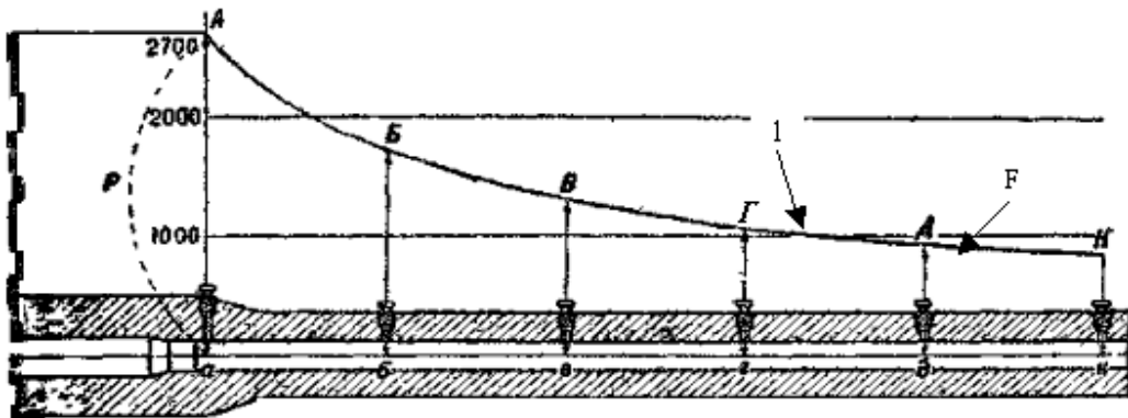
Кривая давления на стенки канала ствола.
