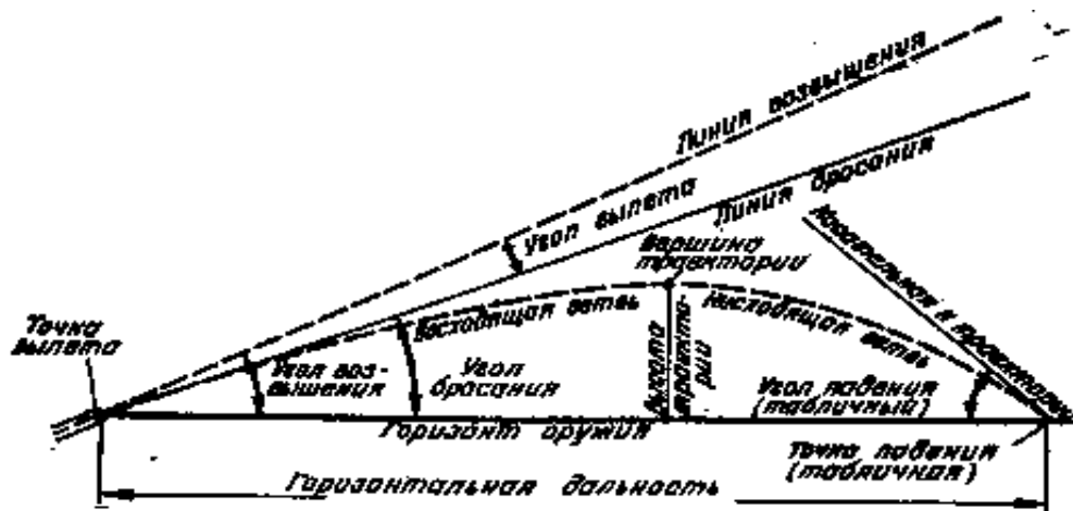
Рис. 49. Элементы траектории полета пули относительно горизонта оружия
