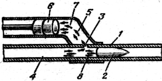
Рис. 46. Принцип работы автоматики:
